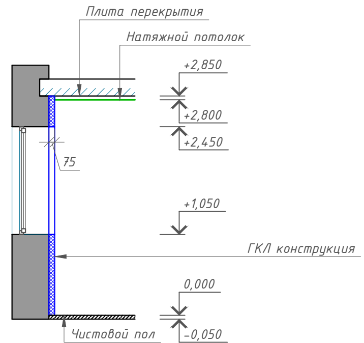
Сечение 1-1
